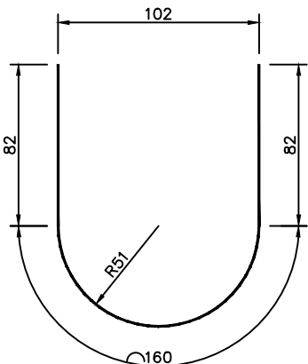
STRAP 1.5 mm G.I
