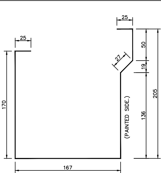
EAVE GUTTER (EG)
