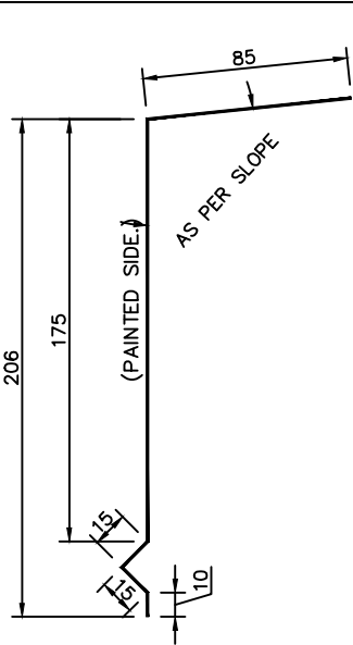
EAVE TRIM (ET)
